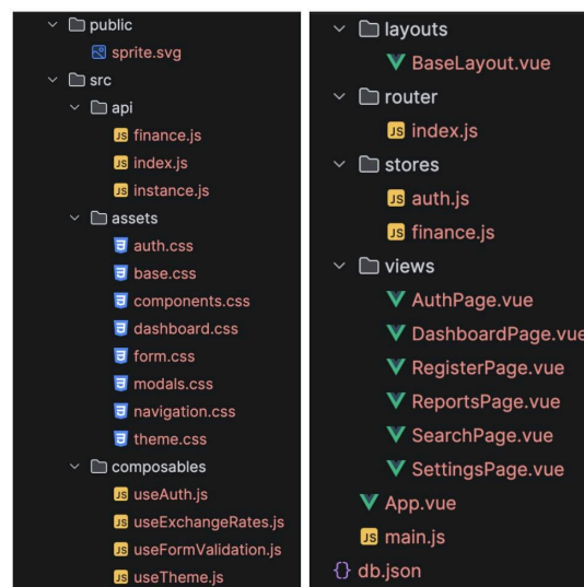
Рис.1. Файловая структура проекта на Vue.js
